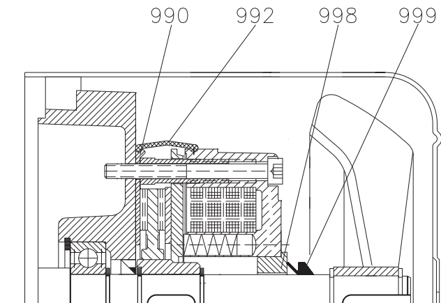
Bremse, Schutzart IP 55, für 5, 10, 20 und 40 Nm Brake, Enclosure IP 55 for 5, 10, 20 and 40 Nm Frein, protection IP 55 pour 5, 10, 20 et 40 Nm
