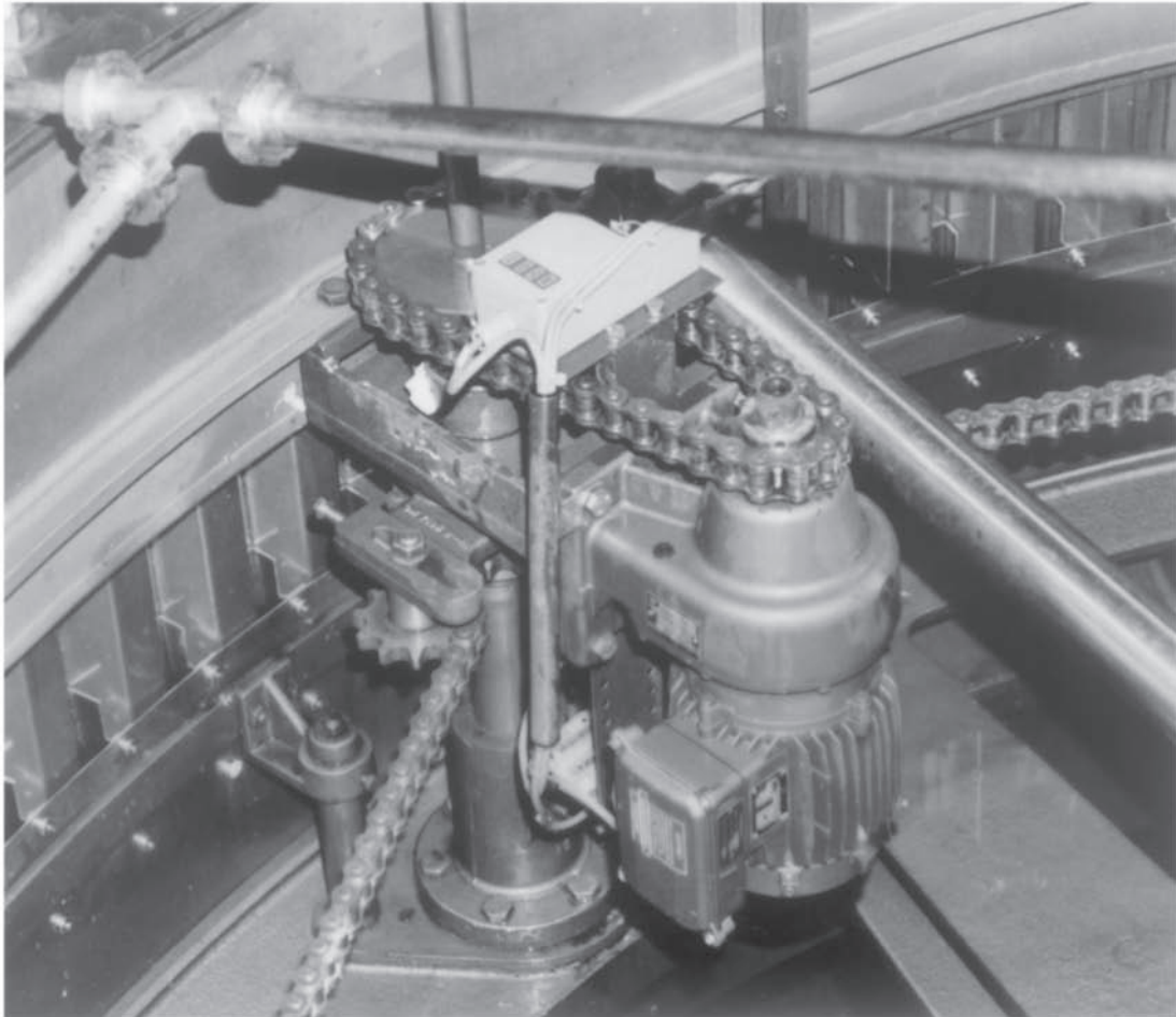
NORD-Stirnradtriebemotor als Antrieb eines Sortierwerkes einer Verschleißmaschine in der Getränkeproduktion NORD-helical geared motor as drive for a sorter-mechanism on a capping-unit in the bottling industry Motoréducteur à engrenages cylindriques NORD pour entraînement d'une capsuleuse en sortie de machine d'embouteillage
