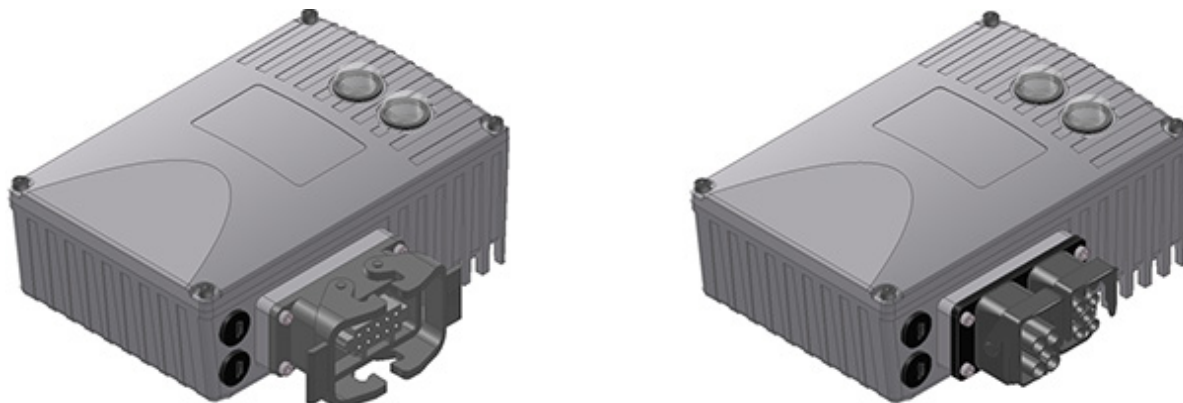
Abbildung 9: Beispiele für Geräte mit Steckverbinder für Leistungsanschluss
